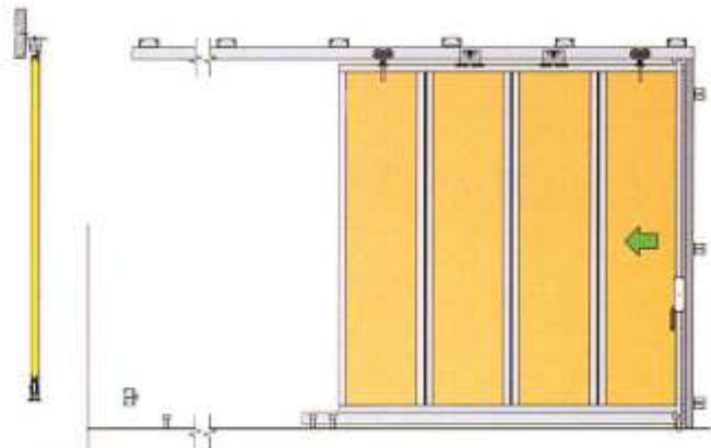
Aplicación de puerta corredera suspendida por un carril superior
